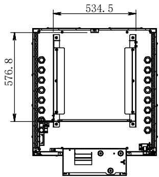
剖面 A-A
