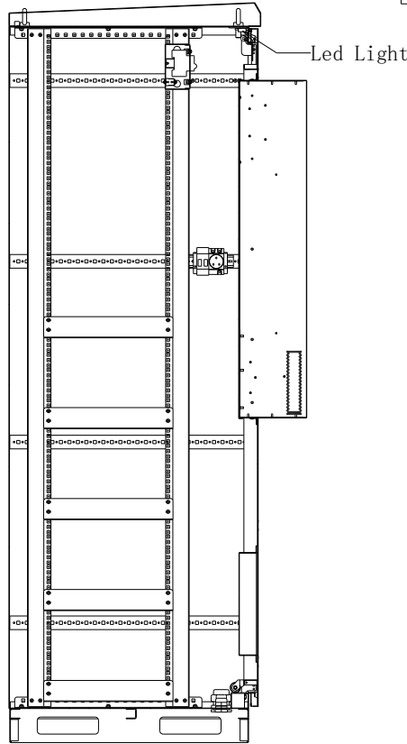
截面 B-B
